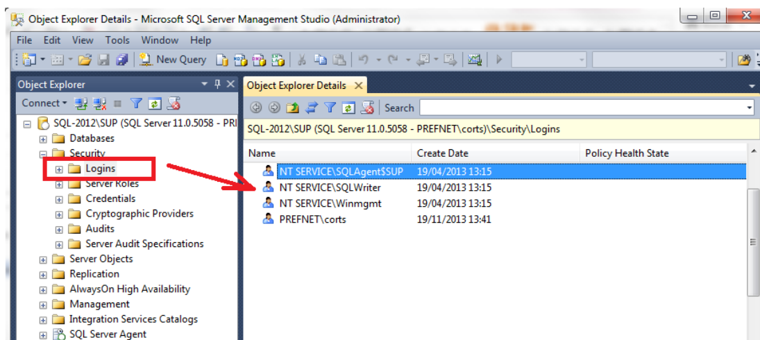
Figura 5. Lista de usuarios dados de alta en SQL Server 2012.
