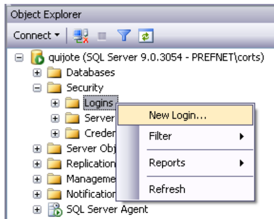
Figura 3. Crear un nuevo inicio de sesión.
