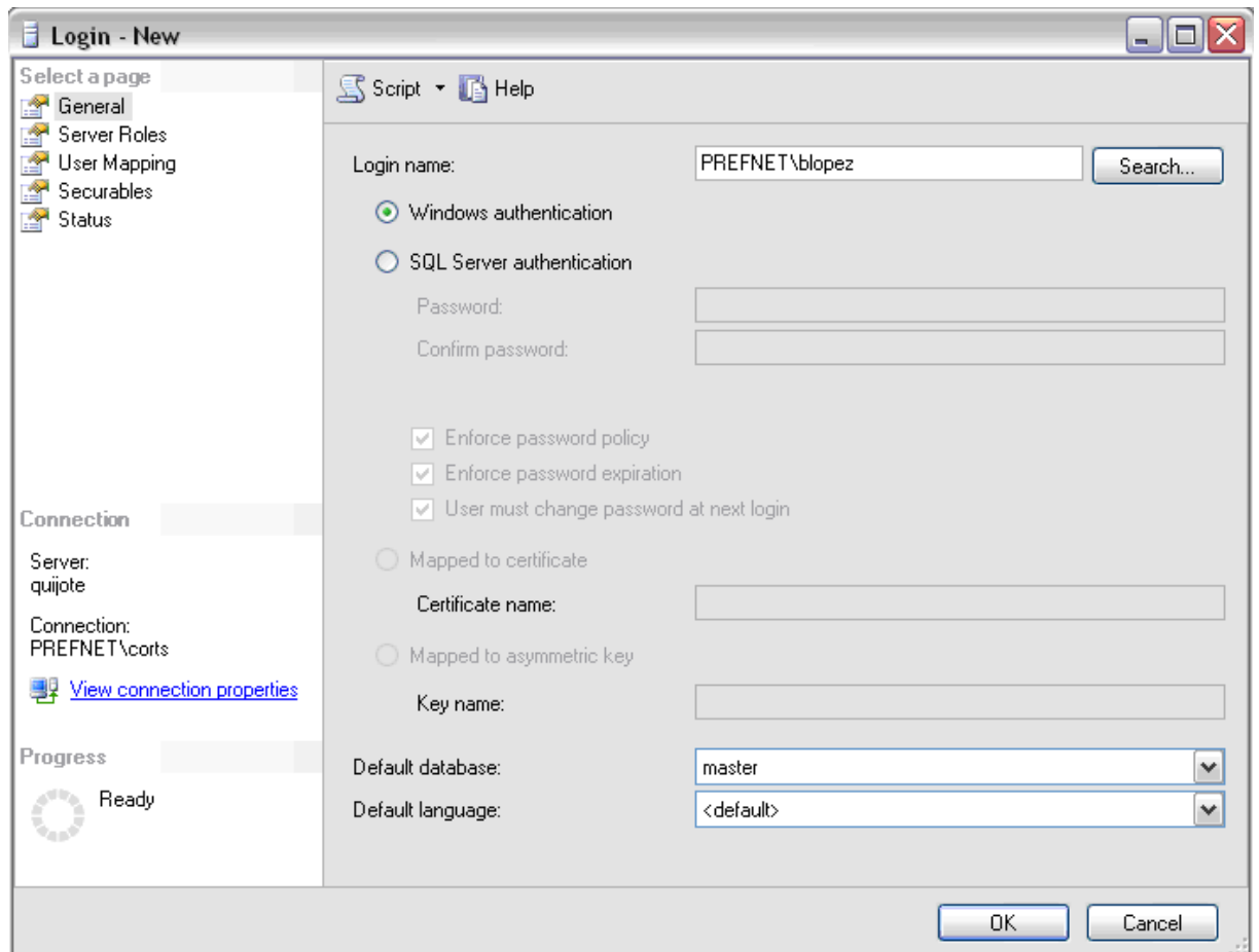
Figura 4. Pantalla “Usuario - Nuevo” o “Login – New”.
