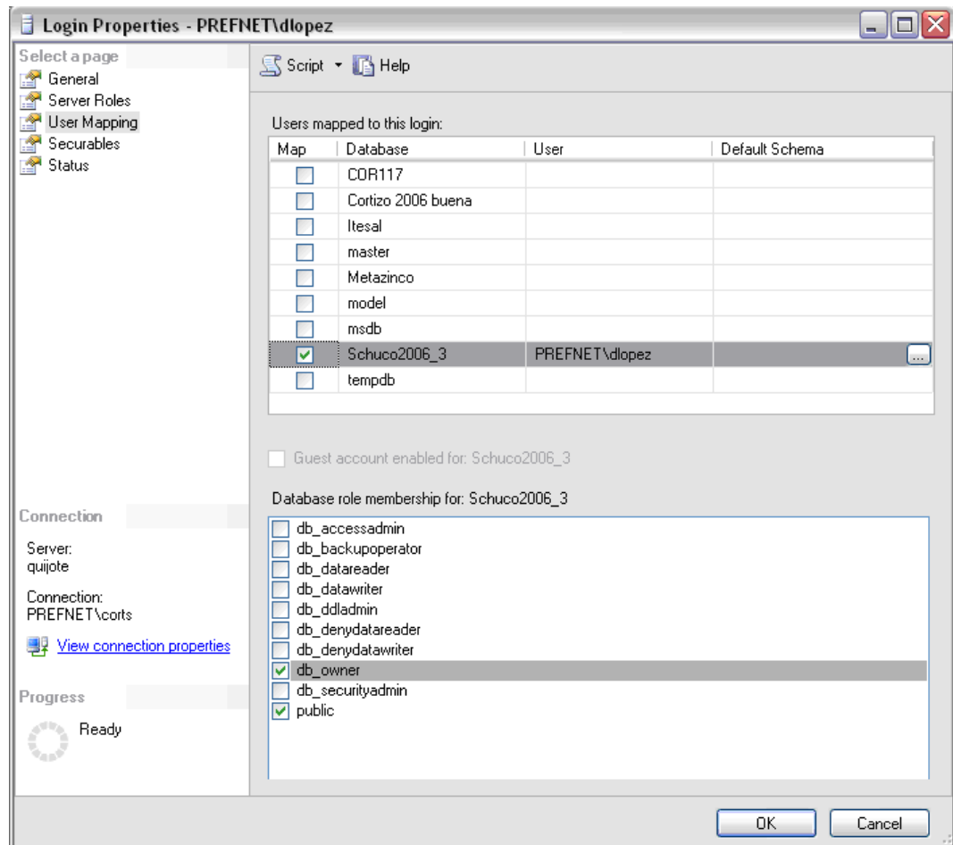
Figura 6. Otorgar permisos de propietario a un usuario en la BD deseada.
